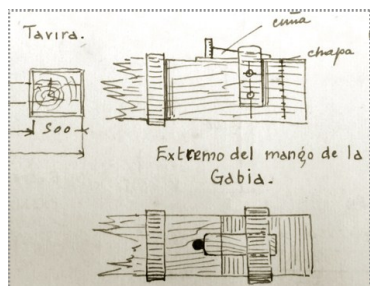
→ Ferrería de Aranekola o Tabira (Durango). Detalle del mazo, dibujo de 1919.
